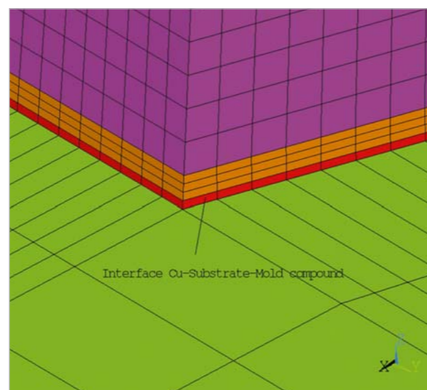
Fig. 3: Interface layer (cohesive zone)
